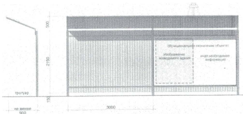
Тип 1.1. Строительное ограждение с навесом
